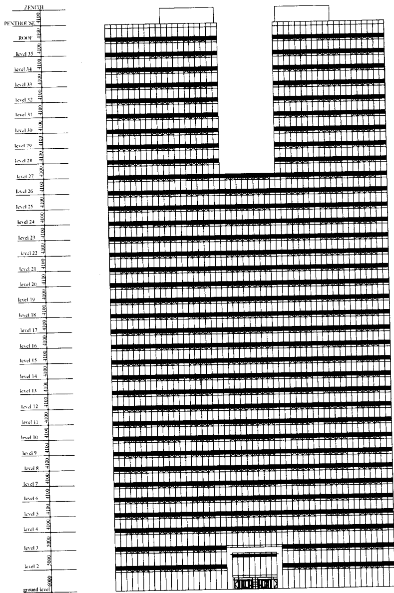
图 25 立面图
