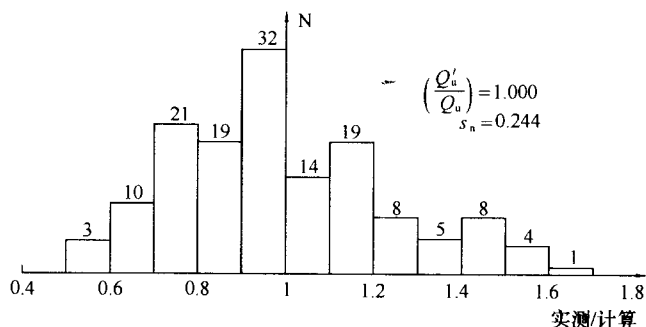
图 13 干作业钻孔桩(144 根)极限承载力实测/计算频数分布
